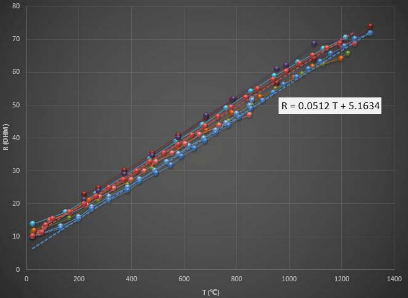
TBC (曹) 热电阻 (R8) 高温特性曲线
